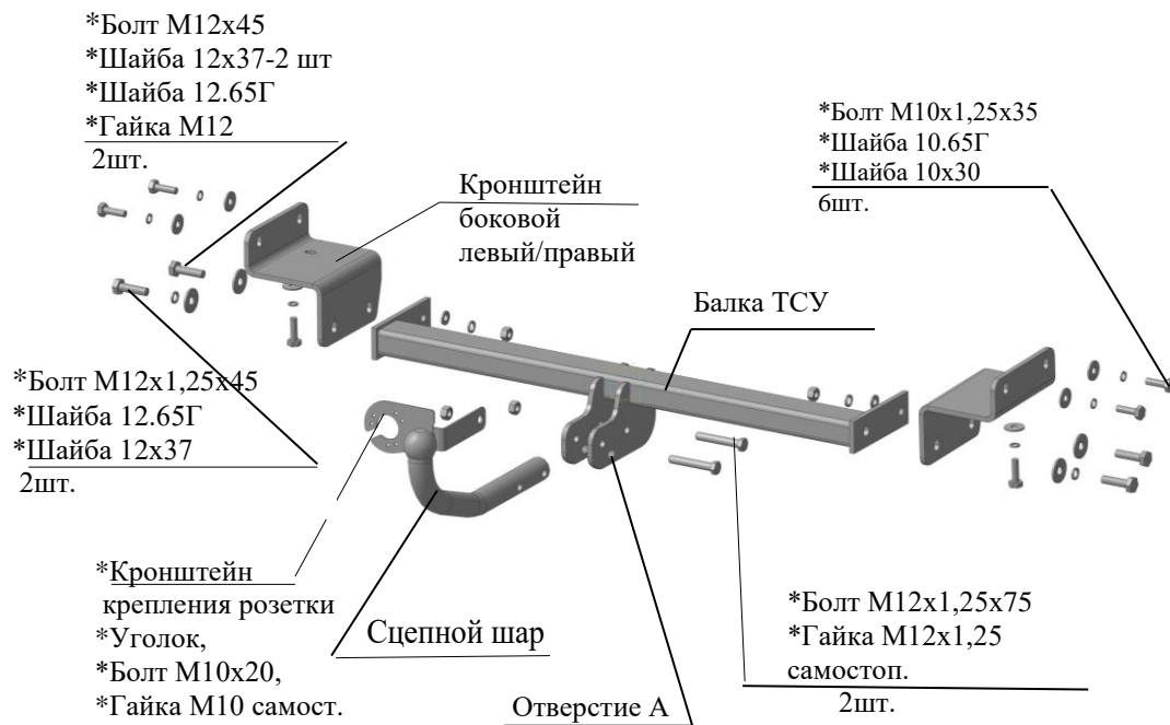
Рис.1 Тягово-сцепное устройство ТСУ 7252.
